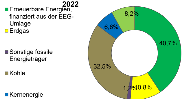
Gesamtenergieträgermix Deutschland 2022
